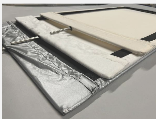
Les Half-Socks conçus en partenariat avec TRP font de vos cadres de drapeaux des supports de tous vos besoins en négatif comme en réfléchi. Adaptables sur gammes TRP, Matthews et Avenger.
